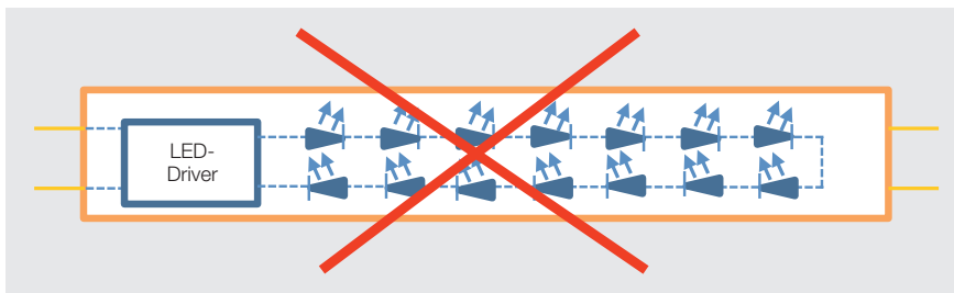
Bild 4 Falsch: Diese Konfiguration ist in der Schweiz verboten. Eine innere Verbindung der leeren Anschlüssen ist Pflicht, sonst kann die LED-Röhre nicht als Retrofit-Lösung für eine Armatur mit KVG verwendet werden.
